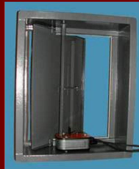
Клпан дымоудаления КДФ-1 с падающей створкой
